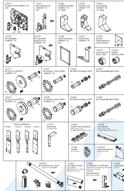
VEKAVARIANT 175 Profilübersicht
