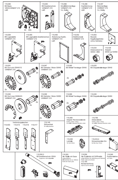
VEKAVARIANT 210 Profilübersicht
