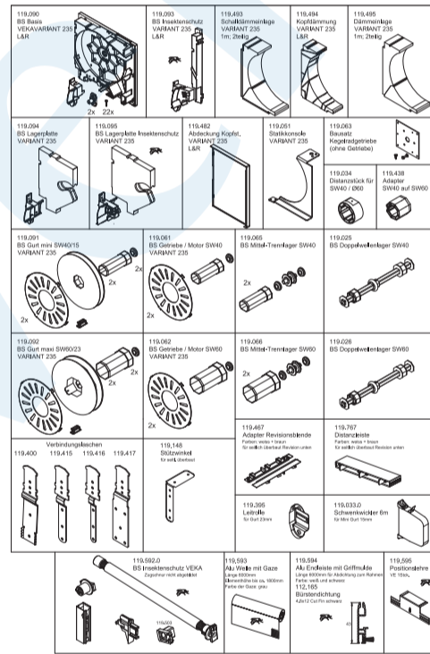
VEKAVARIANT 235 Profilübersicht
